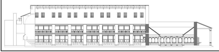
Ek 21. Boyuna Kesit
