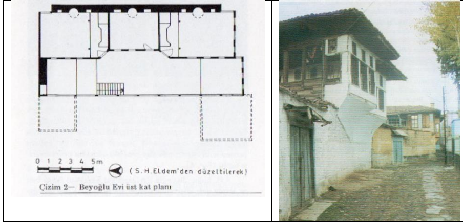
Görsel 8. Beyler evi planı ve sokak görünüşü (Bozer, 1988, 18).
