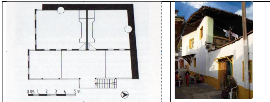
Görsel 11. Külkömür evi planı ve sokak görünüşü (Bozer, 1988, 24).
