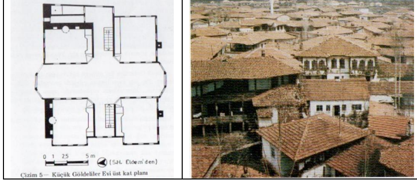
Görsel 12. Küçük gödeliler evi planı ve sokak görünüşü (Bozer, 1988, 32).
